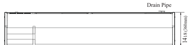
SAKURA-70R / SAKURA-70L TOP VIEW
